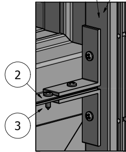
DETAIL A-2
